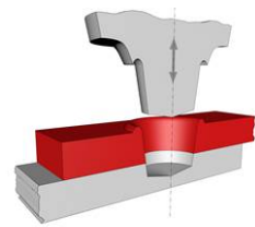
puntlassen
