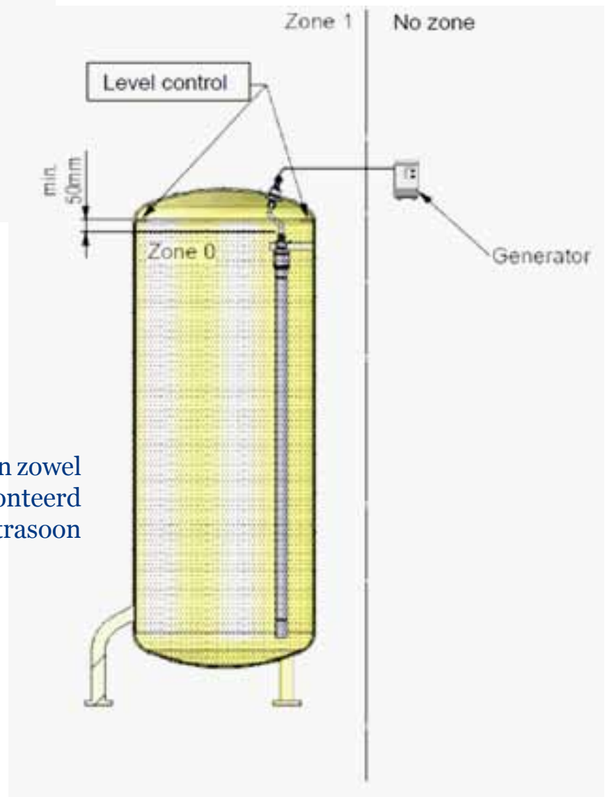
Ultrasoon staafresonator met flens voor zone-afschieding
